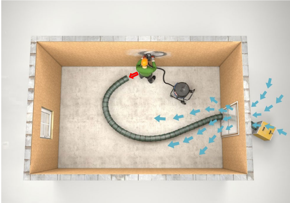
Abbildung 2: Absaugung direkt am Arbeitsplatz mit ergänzendem Einsatz eines Luftreingers
